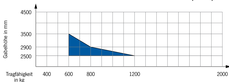
Modell EGV PSL 12-25/12-29/12-35
