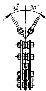
Erlaubter Schrägzug bis Modell TAG 2,0
