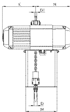
Modell CPV/CPVF mit Aufhängebügel, 250 - 1.000 kg, einsträngig
