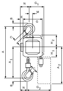
Modell CPE/CPEF mit Traghaken, 1.600 - 3.000 kg, einsträngig
