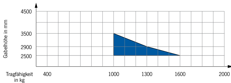
Modell EGV PSH 16-25/16-29/16-35
