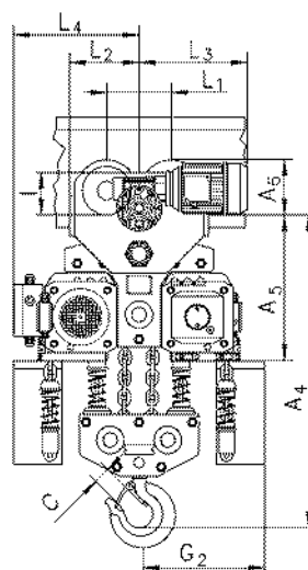
Modell CPE/CPEF Festverbindung mit Elektrofahrwerk, 10.000 kg
