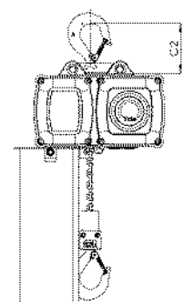
Modell CPV/CPVF mit Traghaken, 250 - 2.000 kg
