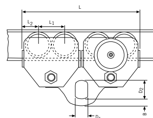
Modell HTG 20.000 kg
