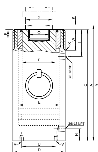
Modell YH-100/50 bis YH 200/500
