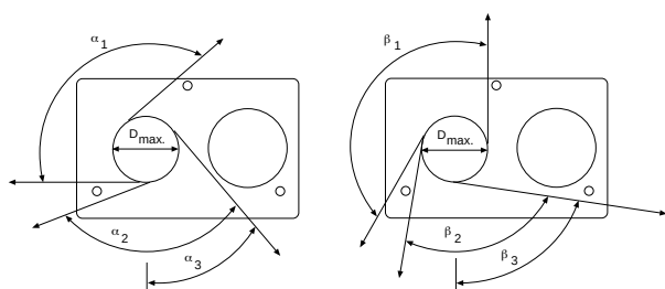
Seilabläufe der Elektroseilwinde Modell RPE
