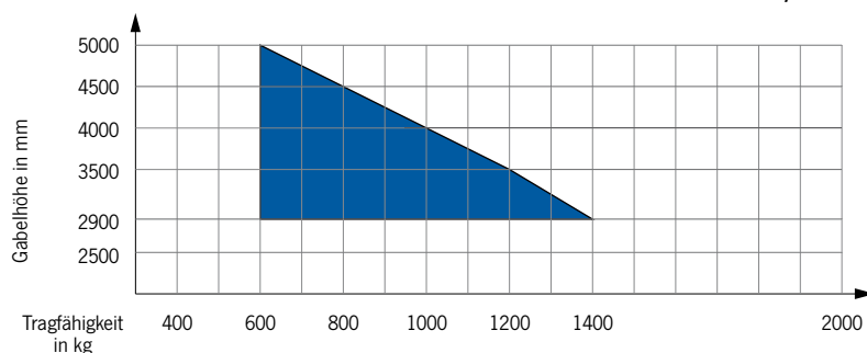
Modell EGV PSH 14-45T/14-50T
