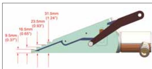
Werkzeug, geschlossen
