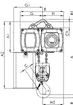
Modell CPV/CPVF mit Aufhängebügel, 500 - 2.000 kg, zweisträngig
