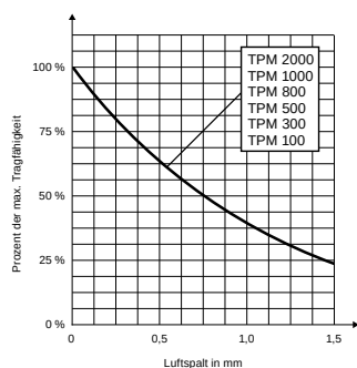
Diagramm: WLL/Luftspalt
