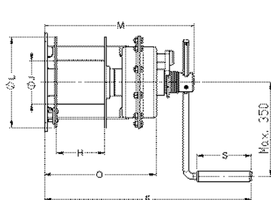
Modell MWS, Traglast 1.000 - 1.500 kg
