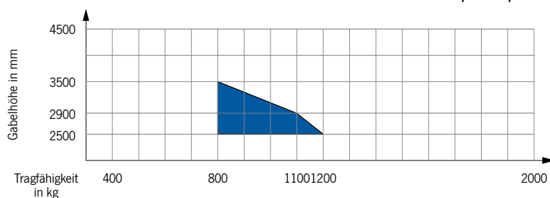
Modell EGV PSH 12-25/12-29/12-35
