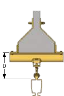
DS Aufhängung für Betonbalken
