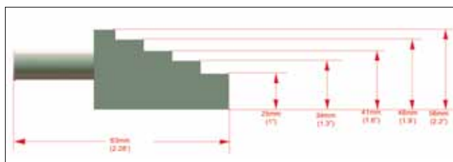
Sicherheitsblock
