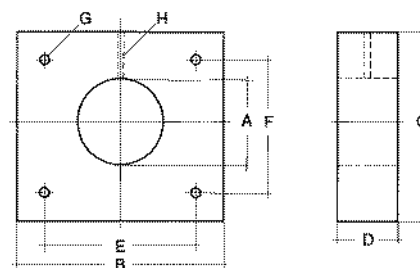
Modell AYP
