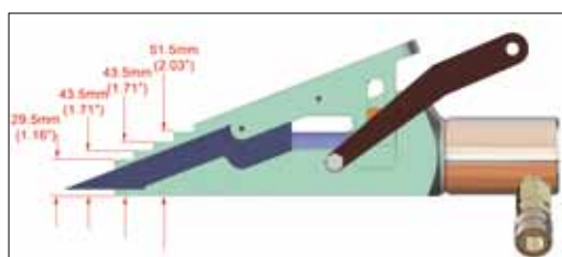
Werkzeug, geöffnet
