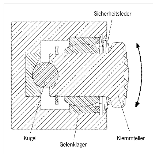
Funktionsskizze Palle
