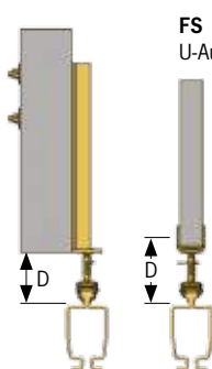
ES Seitenaufhängung
