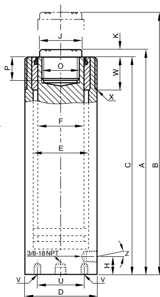
Modell YS-5/25 bis YS-30/200
