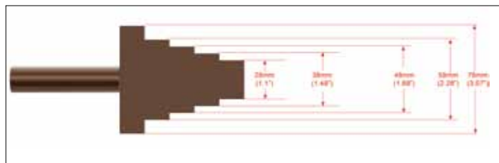
Sicherheitsblock, Seitenansicht
