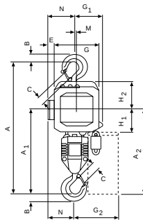
Modell CPE/CPEF mit Traghaken, 3.200 - 5.000 kg, zweisträngig
