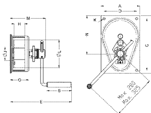
Modell MWS, Traglast 300 - 600 kg
