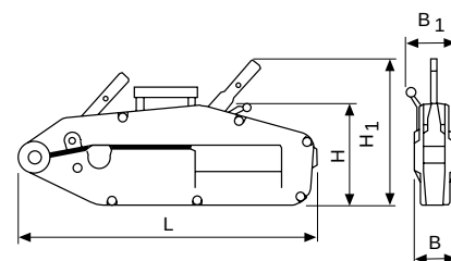
Modell Y 32
