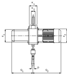
Modell CPE/CPEF mit Traghaken, 1.600 - 3.000 kg, einsträngig
