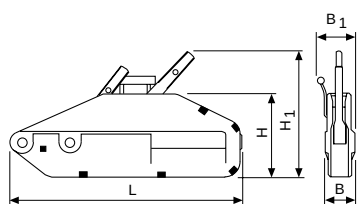
Modell Y 16 ST
