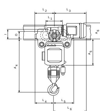
Modell CPE/CPEF Festverbindung mit Elektrofahrwerk
