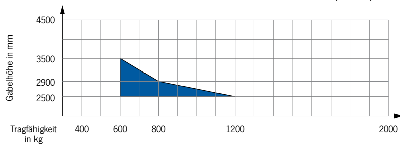
Modell EHH PS 12-25/12-29/12-35
