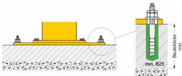
Zwischenfußplatte zum Aufdübeln auf vorhandenem Betonfußboden (nur bei Hallenbetrieb) inkl. Verbundanker HVZ dynamic.
