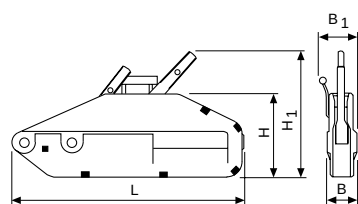
Modell Y 16
