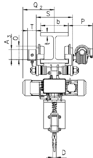
Modell CPE/CPEF Festverbindung mit Elektrofahrwerk, 10.000 kg
