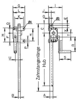
Modell ZWW Tragfähigkeit 1.000 kg
