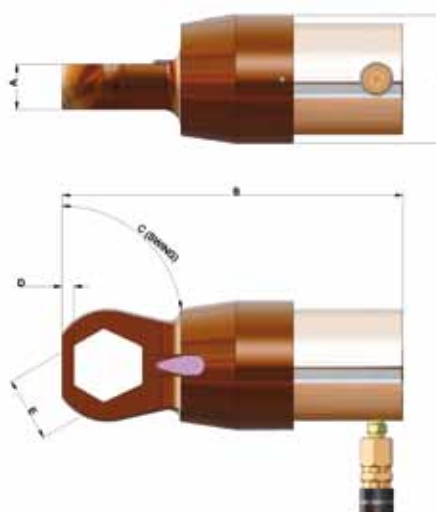
Ausführung Modell YNS
