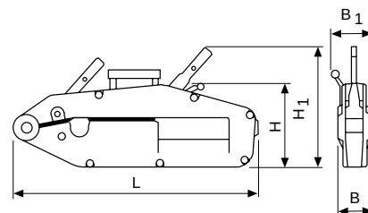
Modell Y 32 ST
