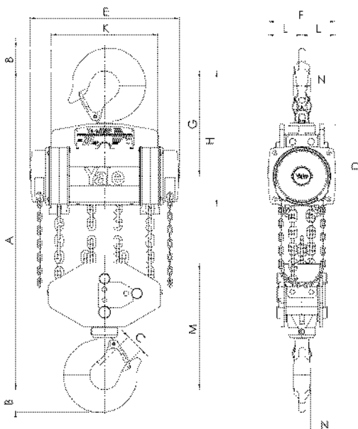
Modell Yalelift 360, 20.000 kg, sechssträngig
