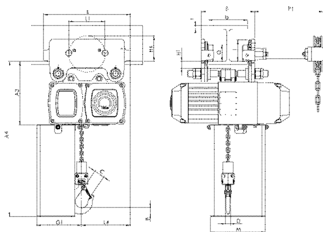
Modell CPV/CPVF Festverbinding mit Roll- oder Haspelfahrwerk
