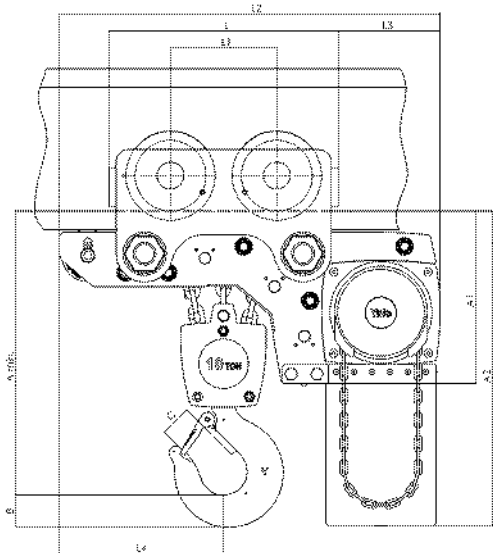
Modell Yalelift LHP/LHG, 10.000 kg, dreisträngig
