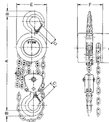
Modell Compact, 500 - 5.000 kg, zweisträngig
