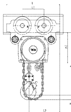
Modell Yalelift ITG, 500 - 3.000 kg, einsträngig
