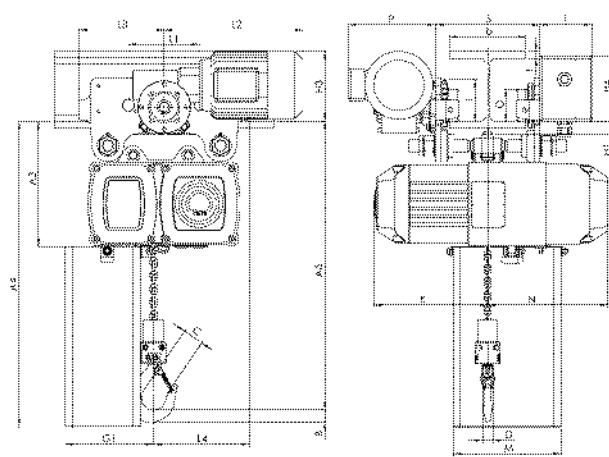
Modell CPV/CPVF Festverbinding mit Elektrofahwerk
