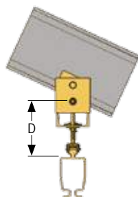
HS Schräge I-Trägeraufhängung
