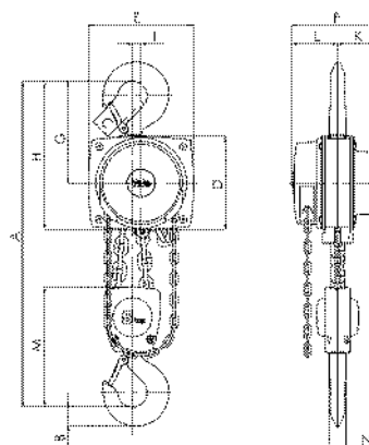
Modell Yalelift 360, 5.000 kg, zweisträngig
