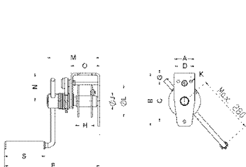
Modell MWS, Traglast 150 kg
