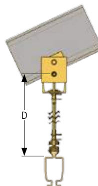
HD Distanzaufhängung für schräge I-Trägeraufhängung
